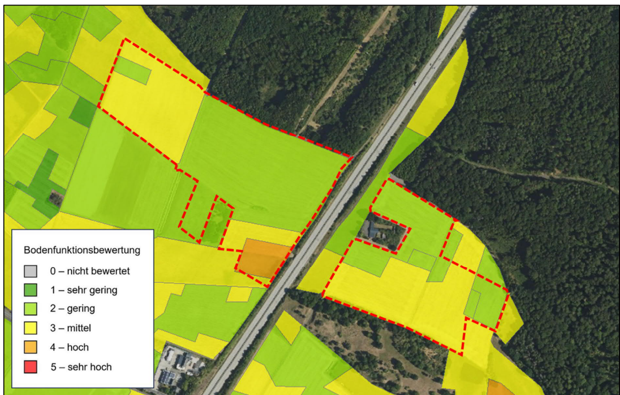
Abb. 2: Bewertung auf Grundlage der Bodenfunktionsbewertung innerhalb des Plangebietes (rot umrandet) sowie der Umgebung (Quelle: BodenViewer Hessen, Zugriff: 16.01.2026, eigene Bearbeitung).
