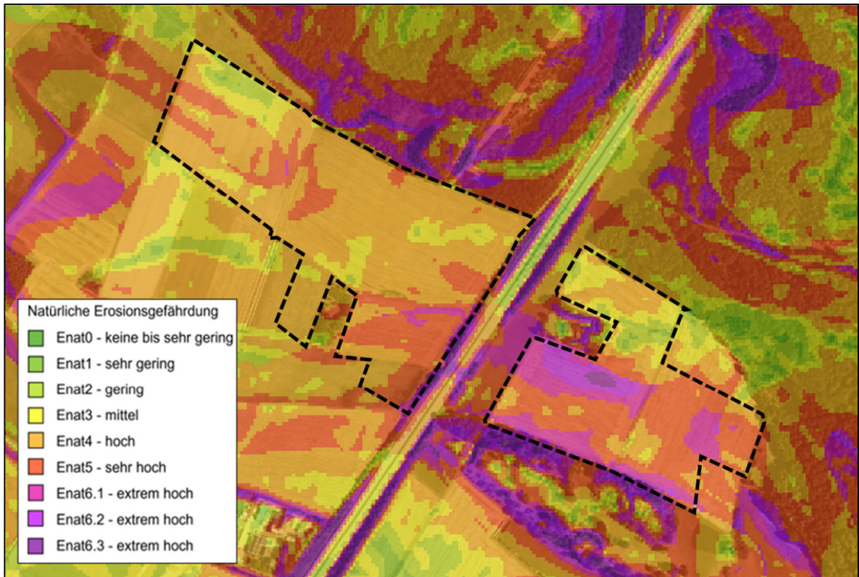
Abb. 3: Natürliche Erosionsgefährdung gemäß Erosionsatlas, Plangebiet: schwarz umrandet (Quelle: BodenVier-Hessen, Zugriff: 16.01.2026, eigene Bearbeitung).
